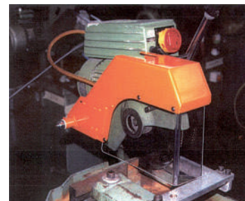
Protección para tronzadora
